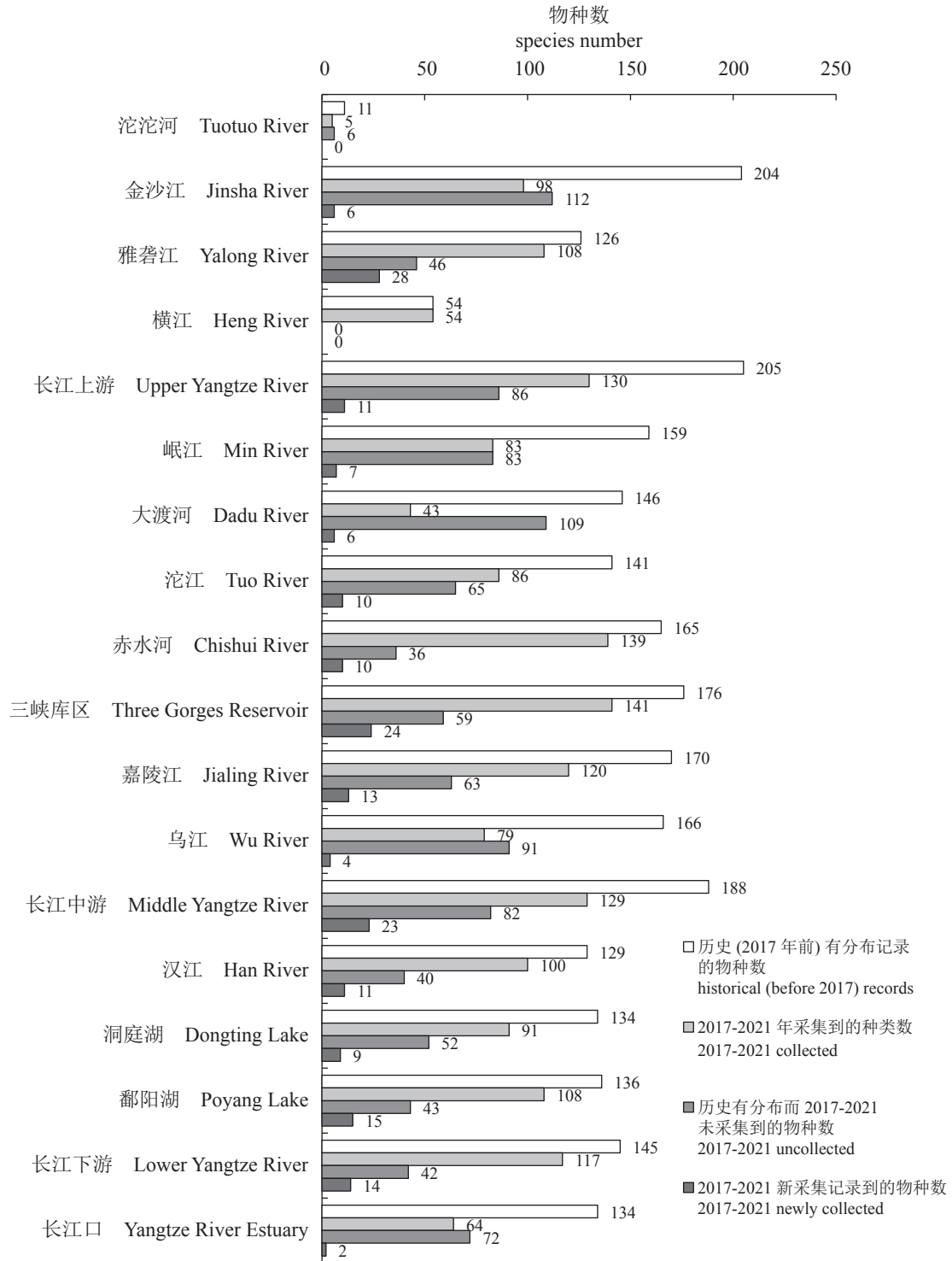
图 2 长江 2017—2021 年鱼类物种采集数量的空间分布
