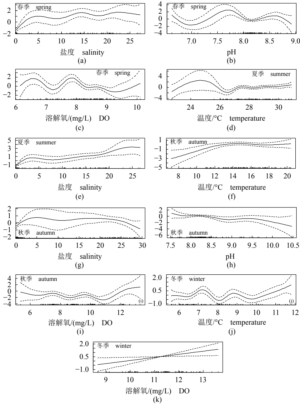
图 2 各季节最佳GAM中环境因子与鱼类资源密度的关系
