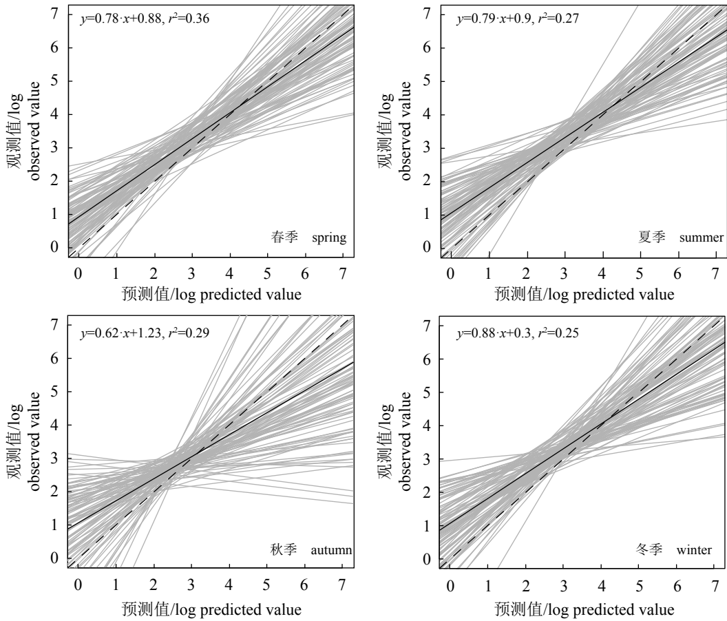
图3 各季度GAM的交叉验证线性回归
