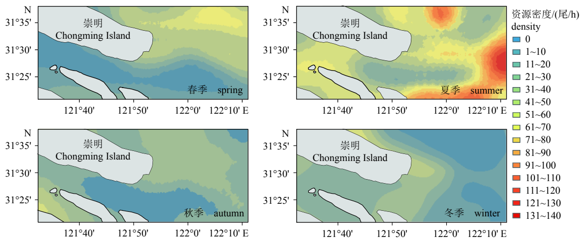
图4 2017年各季度鱼类资源密度预测值空间分布
