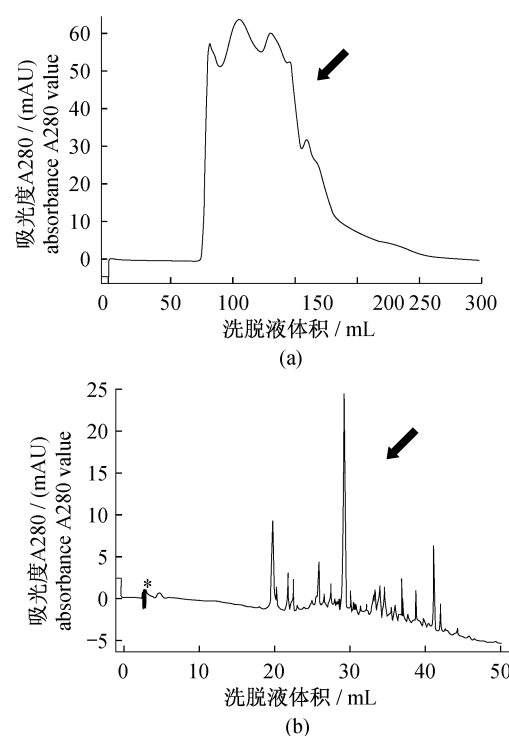
图3 凝胶过滤层析柱和反相液相层析柱联用对日本鳎肝脏小于 10 ku 蛋白样品分离纯化的效果
