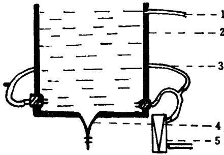
图1 试验水槽装置示意图
